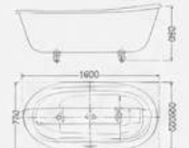
BAÑERA 03715-160 Tamaño: 1600*700*580 mm BAÑERA 03715-170 Tamaño: 1700*705*580 mm BAÑERA 03715-180 Tamaño: 1800*800*580 mm BAÑERA 03715-190 Tamaño: 1900*900*580 mm
